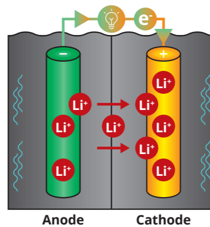
En haut, composants d'une batterie Li-ion. En bas, principe de fonctionnement d'une batterie Li-ion lors de l'utilisation.
